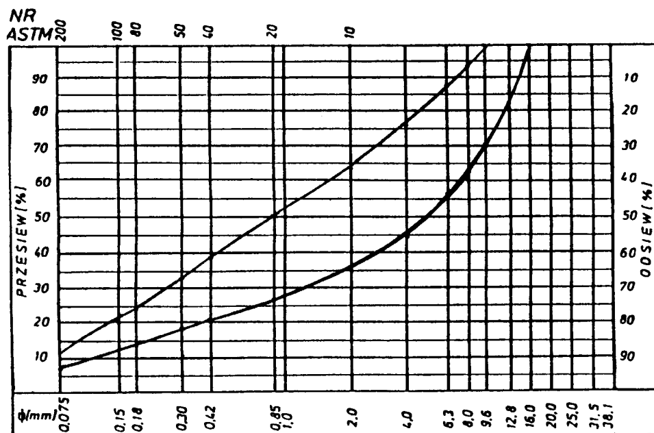
Rys. 1. Krzywe graniczne uziarnienia mieszanki mineralnej 0÷12,8 mm do warstwy ściernalnej z betonu asfaltowego dla KR 3-4
