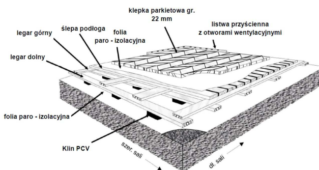
Rys. 1 – Przekrój podłogi sportowej
