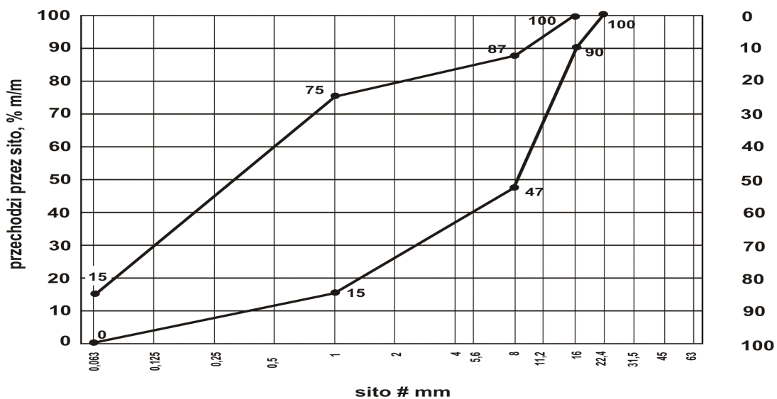
Rys. 3. Uziarnienie mieszanki niezwiązanej 0/16 dla warstwy mrozoochronnej
