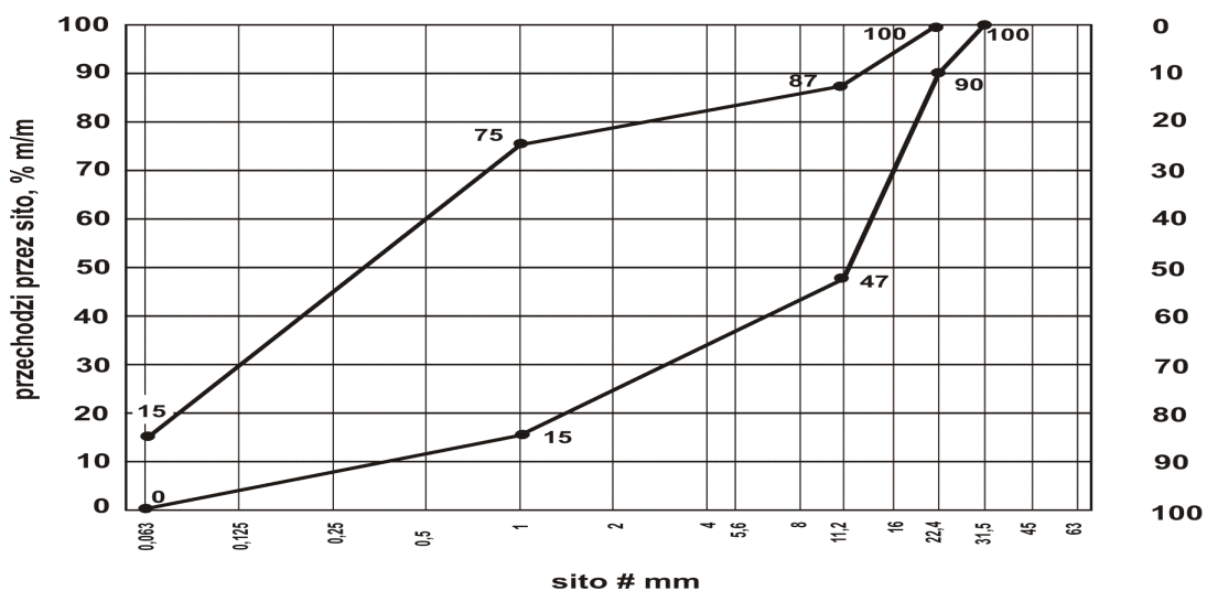
Rys. 4. Uziarnienie mieszanki niezwiązanej 0/22,4 dla warstwy mrozoochronnej
