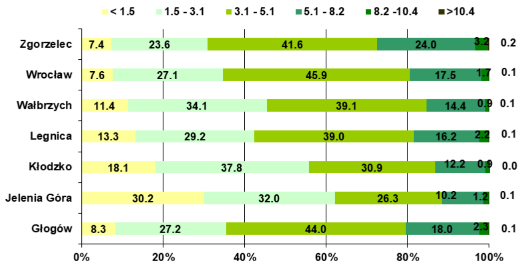
Rysunek 1-23 Częstość występowania prędkości wiatru w określonych przedziałach, w województwie dolnośląskim w 2018 r.
