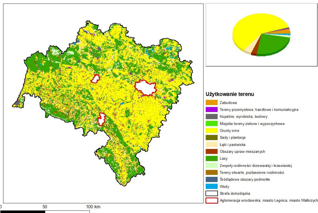
Rysunek 1-16 Użytkowanie terenów w strefie dolnośląskiej
