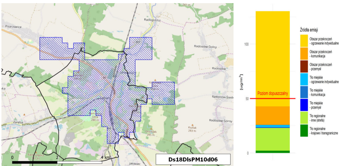
Rysunek 1-52 Obszar przekroczeń średniodobowego poziomu dopuszczalnego pyłu zawieszonego PM10 Ds18DlsPM10d06 w strefie dolnośląskiej, w gminie miejskiej Luban i gminie wiejskiej Luban w 2018 r. wraz z udziałami źródeł emisji w maksymalnych stężeniach na obszarze przekroczeń
