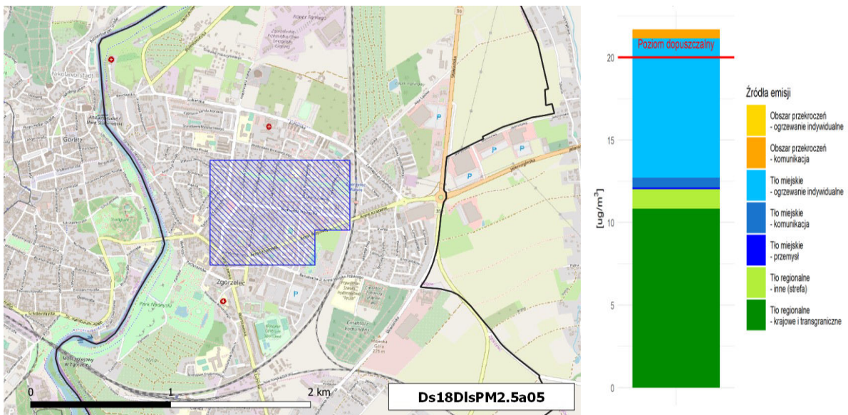
Rysunek 1-67 Obszar przekroczeń poziomu dopuszczalnego pyłu zawieszonego PM 2,5 (faza II) Ds18DIsPM2,5a05 w strefie dolnośląskiej w gminie miejskiej Zgorzelec, w 2018 r. wraz z udziałami źródeł emisji w maksymalnych stężeniach na obszarze przekroczeń
