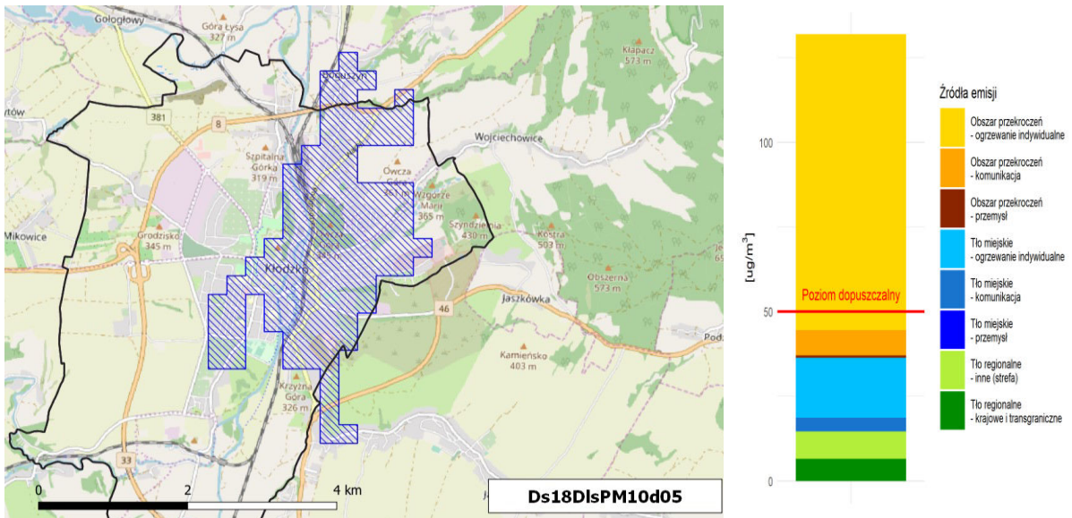
Rysunek 1-51 Obszar przekroczeń średniodobowego poziomu dopuszczalnego pyłu zawieszonego PM10 Ds18DlsPM10d05 w strefie dolnośląskiej, w gminie miejskiej Kłodzko i gminie wiejskiej Kłodzko w 2018 r. wraz z udziałami źródeł emisji w maksymalnych stężeniach na obszarze przekroczeń
